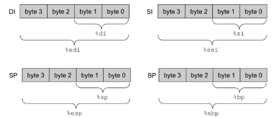
Figura 2.13: Registri IA32
